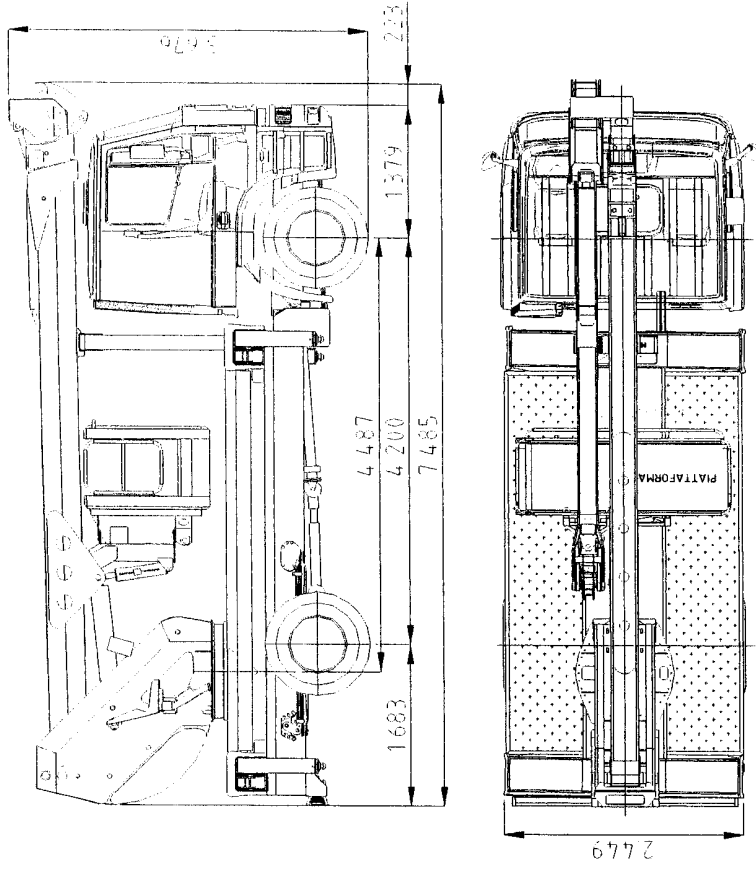
Figura 2: installazione PLE su Iveco EuroTech (cod.K.49.0.0.0.0)
